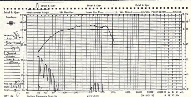
Fig 5. Mätning snarlik den i fig 4. Samma betingelser, dvs som kurvorna är lagda bör nivån ökas med 10 dB för att korrekt markera differensen mellan distorsions- och signaltagning. Frekvensgången för elementet börjar falla av över 40 Hz, varvid distorsionen ligger 35 dB under signalen vid en spänning (6 V) som är något mindre än den som nominellt krävs för driveffekten. Det gör en distorsionsgrad om 1,8 % vid fullt ut bibehållen nivå och frekvensen 40 Hz. Slutet man till basreflexöppningen sjunker kurvan vid 40 Hz drygt 7 dB samtidigt som distorsionen stiger till 3,5 %. — Lyfter man 7 dB på tonkurvan så kommer den i originalregistreringen gröna tonen — som är ointressant — att stiga 14 dB, den röda med 21 dB. Skillnaden, 14 dB, skall dras från 29 dB och vi får då 15 dB, vilket motsvarar en distorsion om 18 % i stället för de ursprungliga 1,8 procenten. Slutsatsen är alltså att vid en viss ljudnivå uppstår 10 ggr högre distorsion vid en sluten låda än vid en basreflexlösning.
